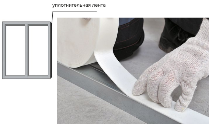
Рис. 3. Схема расположения и приклейка уплотнительной ленты в каркасе
