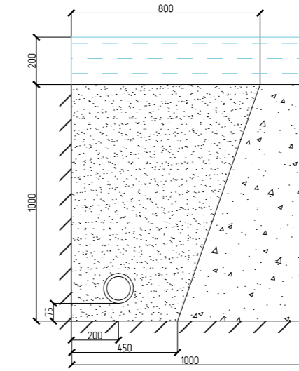
Рис. 1. Классическое решение пристенного дренажа (СССР, 1963 год).
